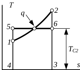
Рис.8.9. К определению среднеинтегральной температуры
