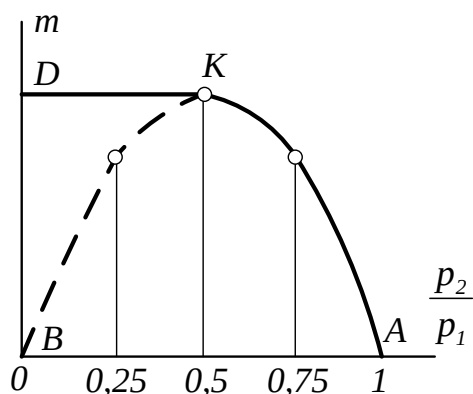
Рис.9.5. Диаграмма расхода газа
