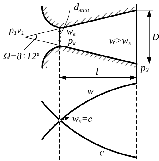
Рис.9.10. Истечение идеального газа из комбинированного сопла Лавая
