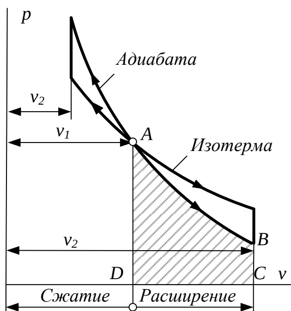
Рис. 7.6. Сравнение адиабаты и изотермы на p - v диаграмме
