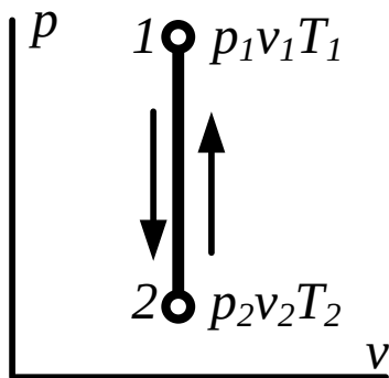
Рис. 7.1. Изохорный процесс на p - v диаграмме
