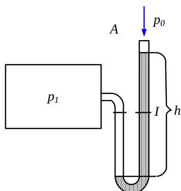
Рис. 1.1. Измерение давления высотой столба жидкости
