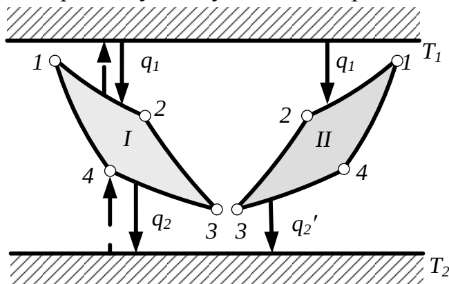
Рис.8.5. К доказательству теоремы Карно
