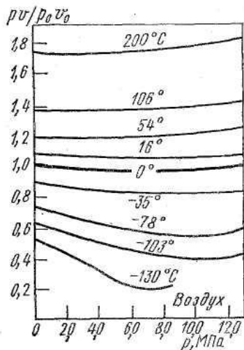
Рис. 4.2. Зависимость от- ношения p \cdot v / (p_0 \cdot v_0) от давления для воздуха
