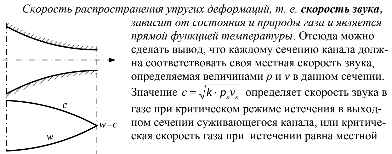
Рис.9.6. Скорость истечения в выходном сечении суживающегося канала
