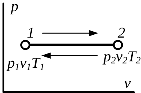
Рис.7.3. Изобарный процесс на p - v диаграмме
