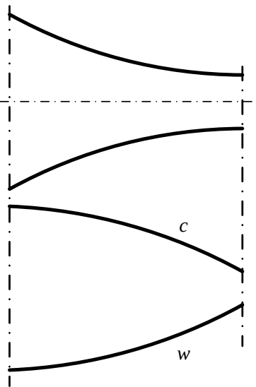
Рис.9.8. Первый случай истечения идеального газа из сужающегося сопла
