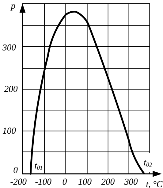
Рис.10.2. Инверсионная кривая для азота T_{ин} = f(p)
