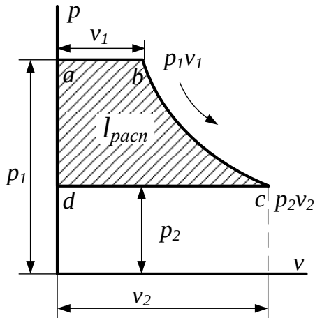
Рис.9.4. Располагаемая работа при истечении газа
