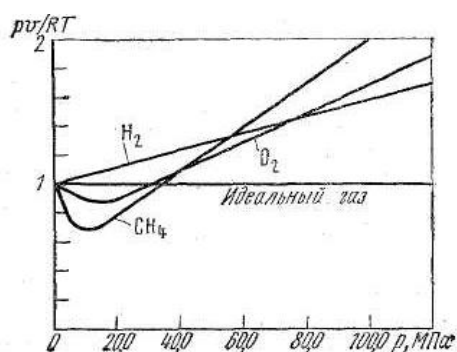
Рис.4.1. Зависимость коэффициента сжимаемости Z от давления при температуре t = 0^\circ\text{C} для некоторых газов
