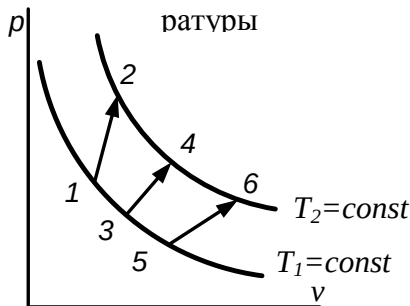
Рис. 5.2. К определению зависимости внутренней энергии от температуры
