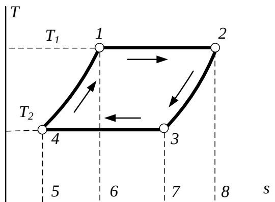
Рис.8.8. Обобщенный (регенеративный) цикл Карно
