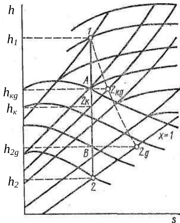
Рис.9.11. Процессы истечения водяного пара
