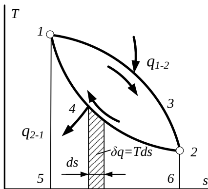
Рис.6.3. Тепловая T - s диаграмма
