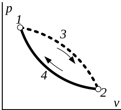
Рис.8.7. К рассмотрению изменения энтропии при необратимых процессах
