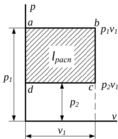
Рис.9.3. Располагаемая работа при истечении капельной жидкости
