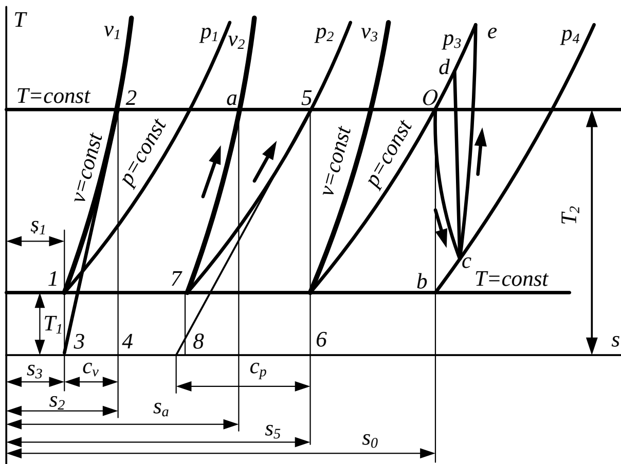
Рис.7.2. Термодинамические процессы на T - s диаграмме
