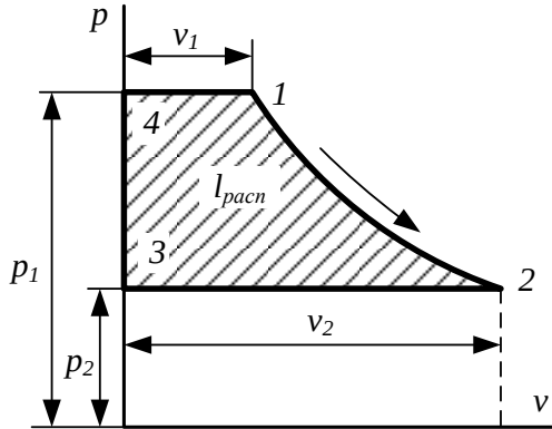
Рис.9.7. Располагаемая работа при истечении идеального газа из сужающегося сопла при \beta_* < p_2 / p_1 < 1
