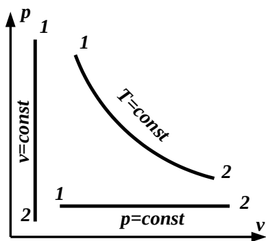
Рис.1.2. Термодинамические процессы в координатах p - v
