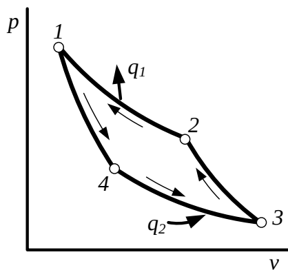
Рис.8.4. Обратный обратимый цикл Карно
