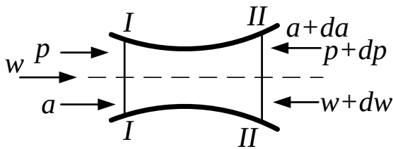
Рис.9.1. Перемещение газа по каналу переменного сечения
