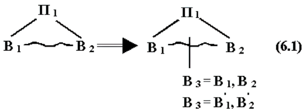
Рис. 6.4. Вепольная структура
