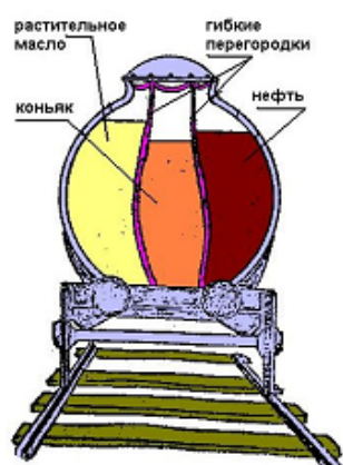
Цистерна с гибкими перегородками
