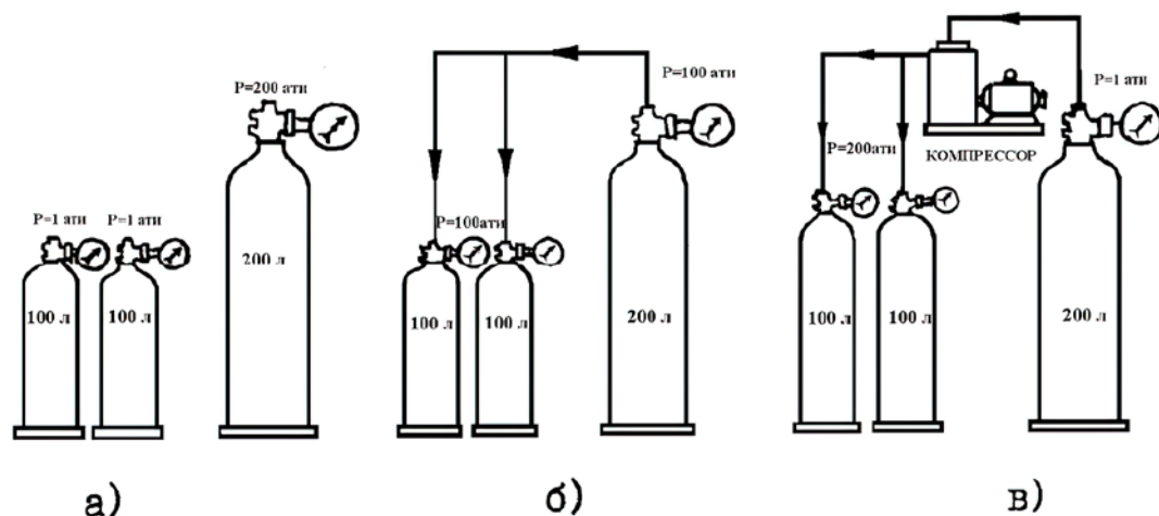
Рисунок 4.1 Перекачка газа
