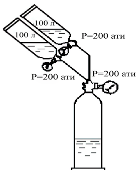
Рисунок 4.2 Перекачка газа (решение)
