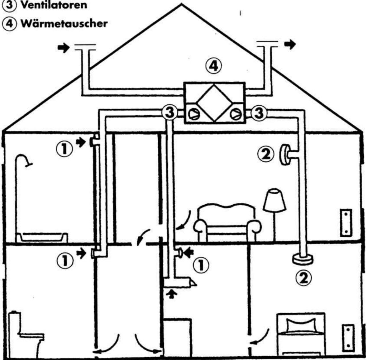
Abb. 11: Wohnungslüftung mit Wärmerückgewinnung.
