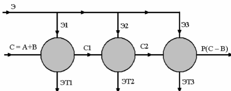
Рис. 6. Схема перекрестно-точной экстракции Обозначение потоков: C – исходная смесь; A и B – компоненты смеси; \mathcal{E} – экстрагент; \mathcal{E}T – экстракт; P – рафинат
