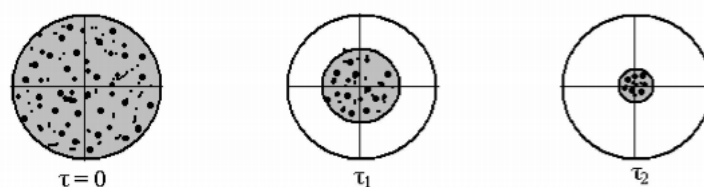
Рис. 9. Изменения состава твердого тела в процессе экстрагирования
