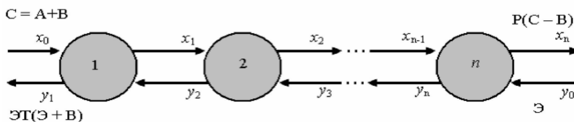
Рис. 7. Схема многоступенчатой противоточной экстракции. Обозначение потоков: С – исходная смесь; А и В – компоненты смеси; Э – экстрагент; ЭТ – экстракт; Р – рафинат
