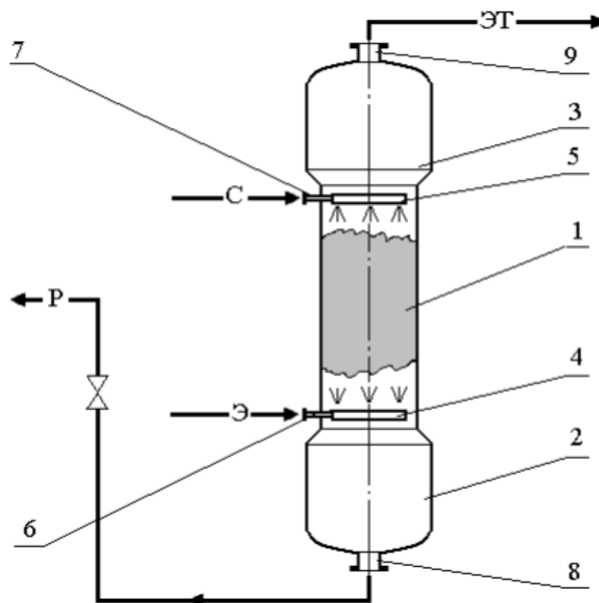
Рис. 8. Гравитационный полный распылительный экстрактор 1 – корпус; 2 и 3 – отстойные зоны; 4 и 5 – распределители легкой и тяжелой фаз. Штуцера: 6 – для подвода легкой фазы; 7 – для подвода тяжелой фазы; 8 – для отвода тяжелой фазы; 9 – для отвода легкой фазы. Потоки: С – исходная смесь; Э – экстрагент; ЭТ – экстракт; Р – рафинат
