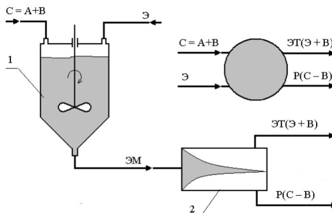
Рис.5. Схема процесса одноступенчатой экстракции
