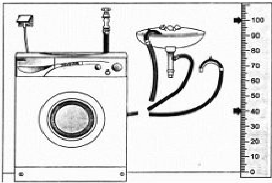
Эргономические параметры подключения стиральной машины
