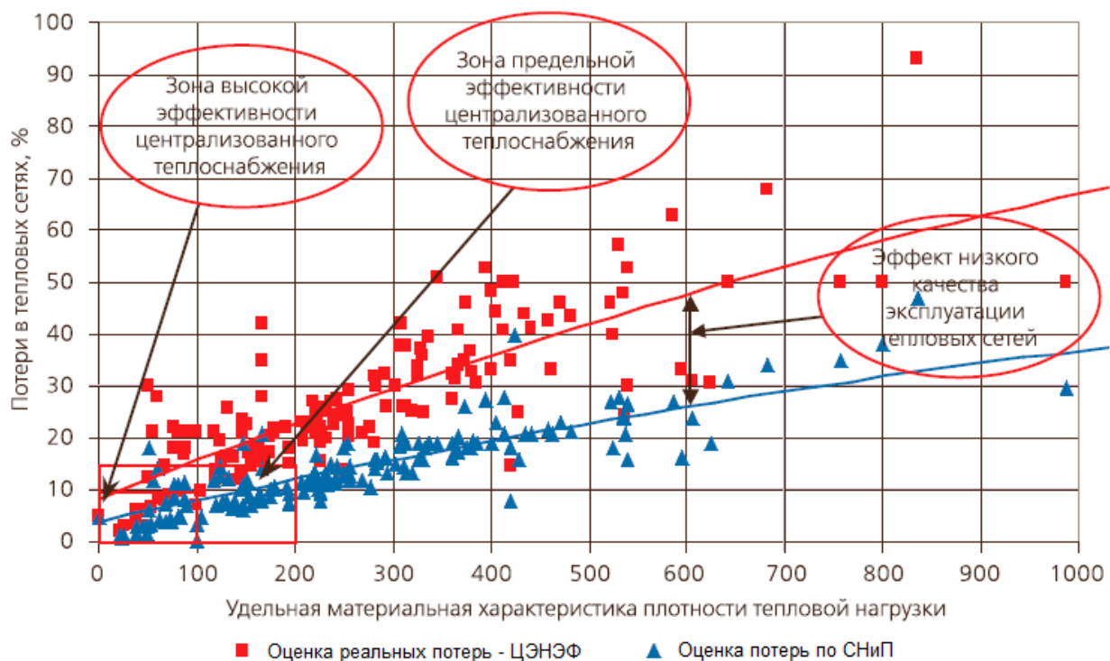
Рис. 1. Потери в тепловых сетях
