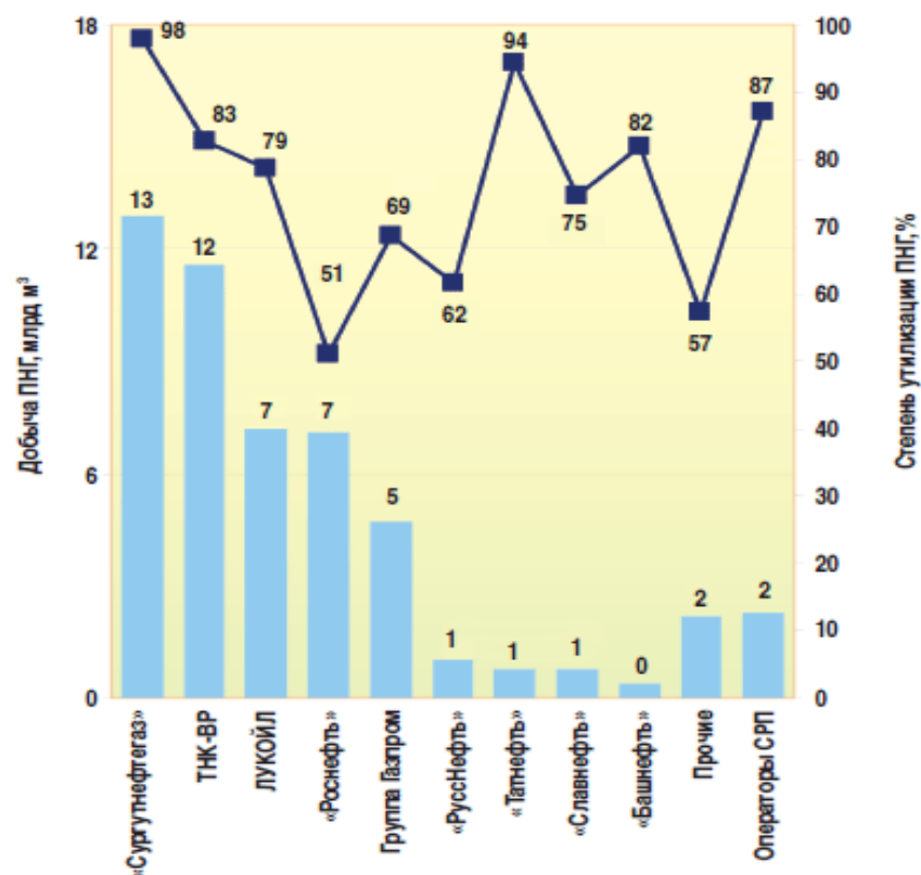
Рис. 2. Добыча и степень эффективного использования ПНГ в России
