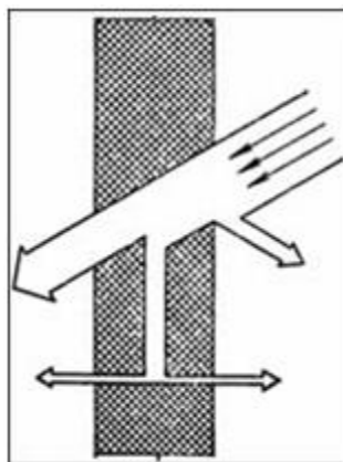
Рис. 10. Схема распределения солнечного теплового потока
