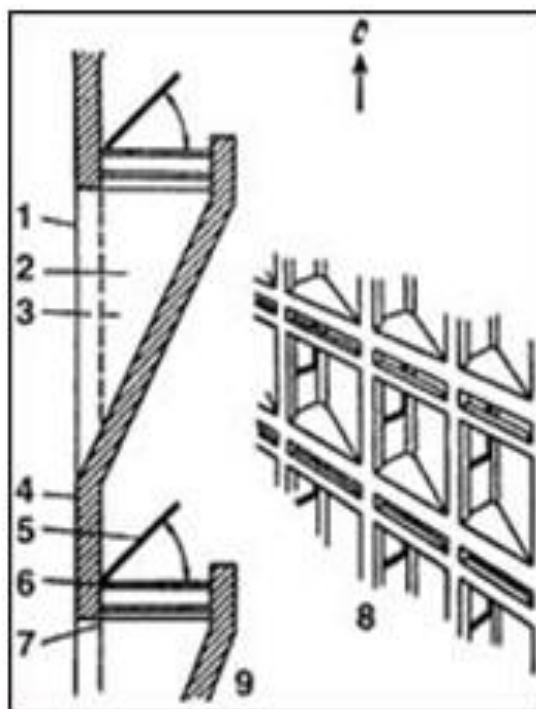
Рис. 12. Пилообразное расположение окон на западном фасаде здания:
