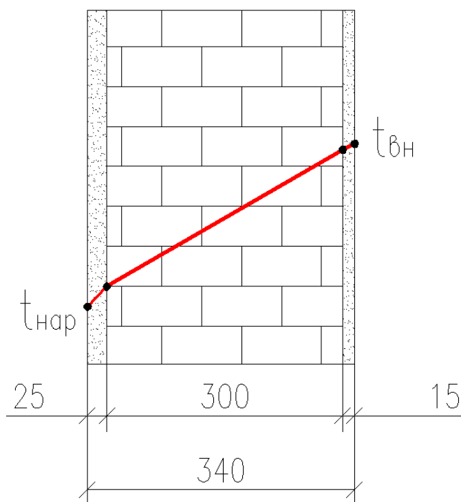
Рис. 35. Кирпичная кладка
