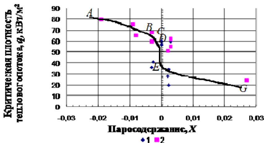
Рисунок 2.9. Зависимость паросодержания от q_{кр} при кипении черной сульфатной щелочи и водного предгидролизата: w_0 = 0,015 - 0,025 м/с; \rho_w = 25 кг/(м 2 с); 1 - B < 30 %; 2 - B > 30 % абсолютно сухих веществ (а.с.в)
