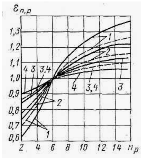
Рисунок 2.5. Значение \varepsilon_{n,p} при кипении фреона-12 на пучке оребренных труб:
