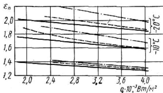
Рисунок 2.3. Зависимость коэффициента \varepsilon_{\text{п}} от плотности теплового потока q , температуры насыщения t_{\text{н}} и относительного шага пучка S/d : S/d = 1,45 ; ---- S/d = 1,3 ; - - - - S/d = 1,15
