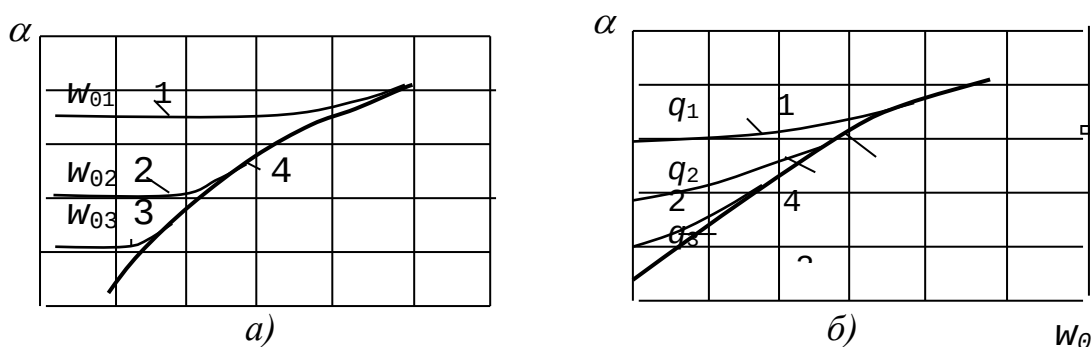
Рисунок 2.7. Качественный характер изменения теплоотдачи при кипении в трубах в зависимости от скорости циркуляции и тепловой нагрузки:
