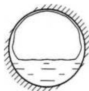
Рисунок 1.6. Изменение структуры парожидкостного потока при конденсации в горизонтальной трубе
