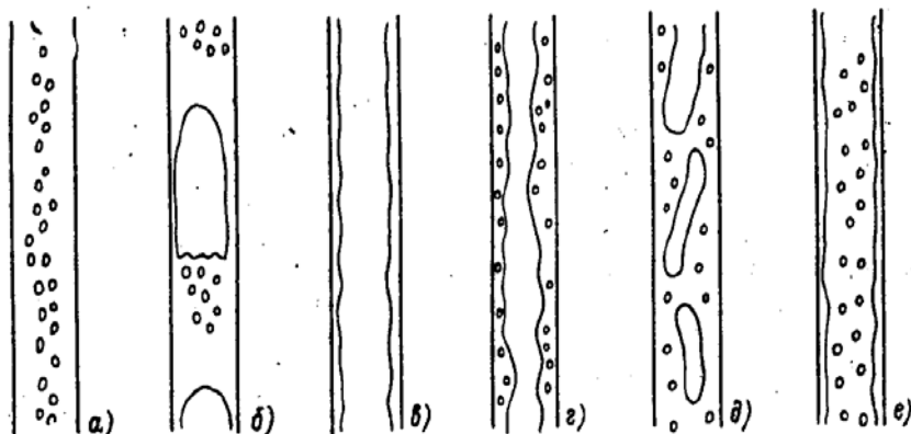
Рисунок 2.8. Нисходящий поток в вертикальной трубе:
