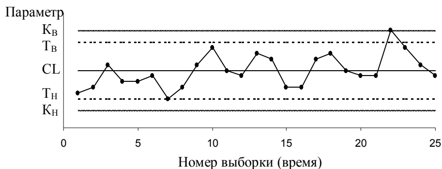
Рис.13.1. Пример контрольной карты
