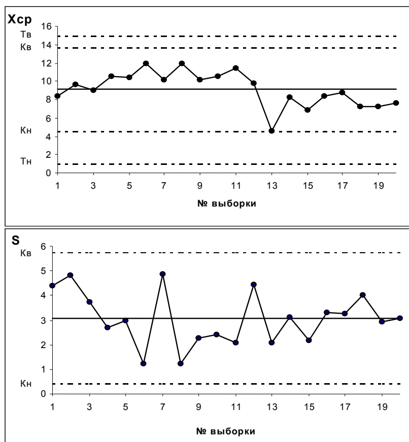
Рис.13.2. \bar{X} –S-карта, полученная в примере
