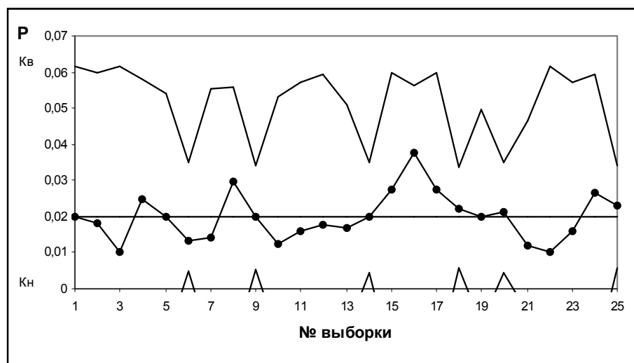
Рис 14.1. Контрольная p-карта по данным табл. 14.1
