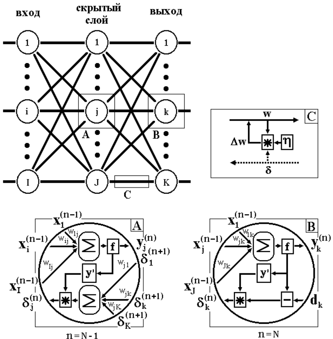
Рис.11. Диаграмма сигналов в сети при обучении по алгоритму обратного распространения ошибки
