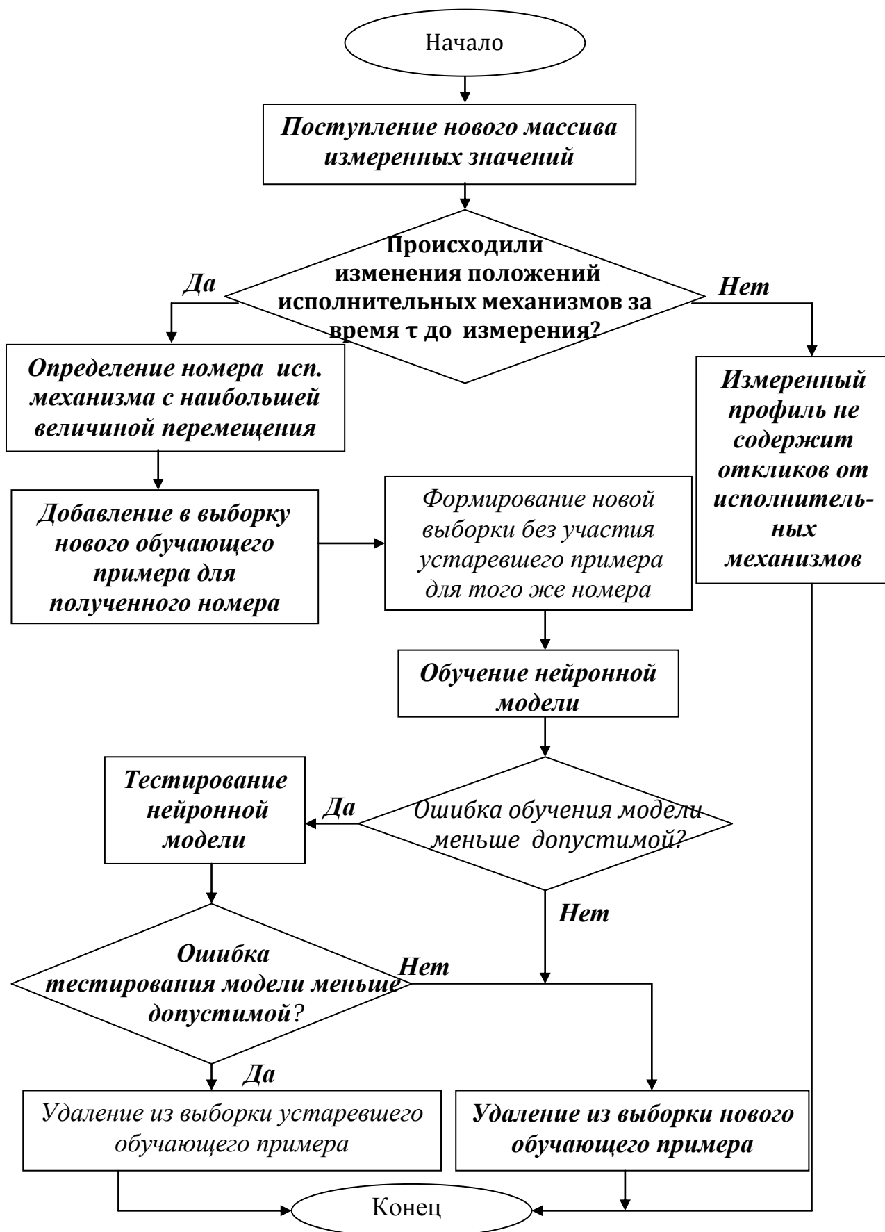
Рис.17. Алгоритм формирования обучающей выборки
