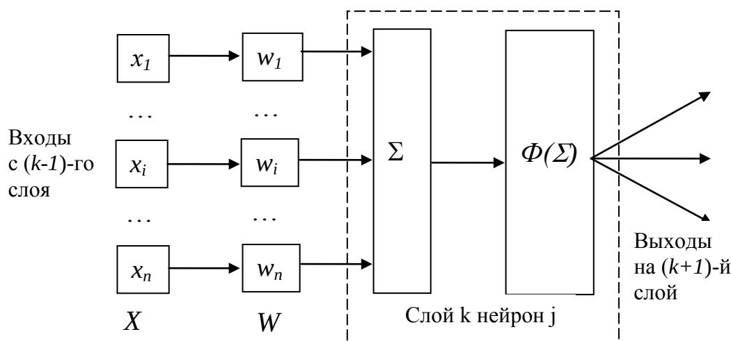
Рис.3. Структура искусственного нейрона
