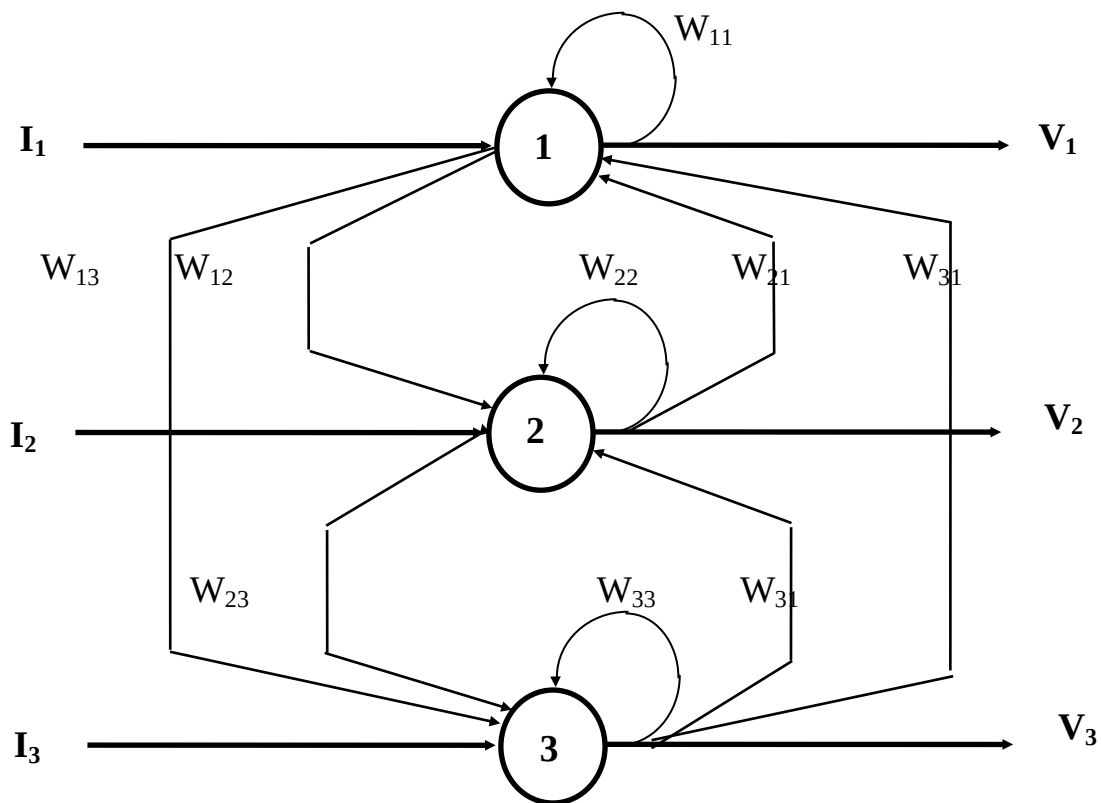
Рис.10. Сеть Хопфилда «Hopfield net» с тремя нейронами
