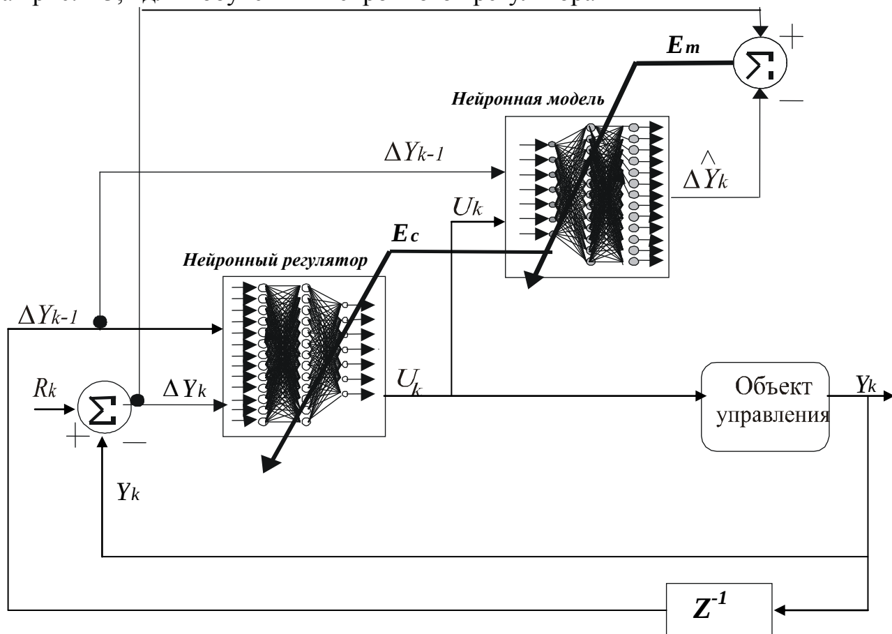
Рис.12. Структурная схема с применением обучаемой нейронной модели объекта для обучения нейронного регулятора
