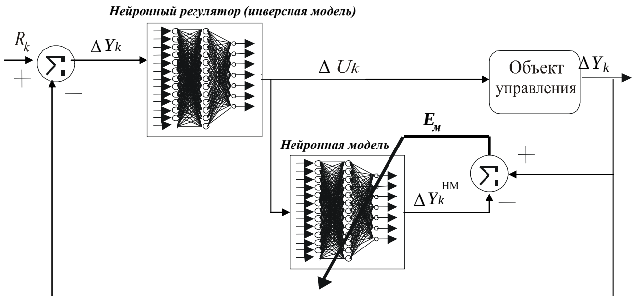
Рис. 14. Структурная схема инверсного использования нейронной модели в качестве регулятора
