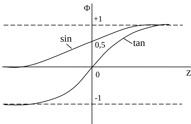
Рис.5. Графики сжимающих функций
