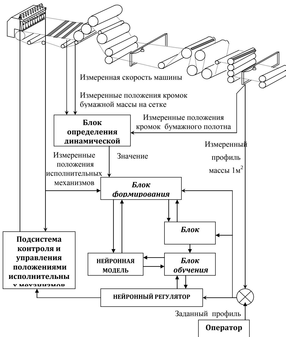
Рис.15. Схема нейросетевой системы управления массой 1 \text{ м}^2 бумаги
