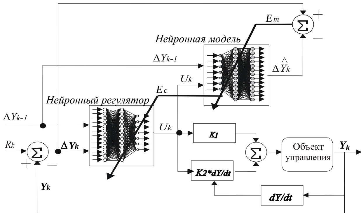
Рис.19. Структурная схема системы управления с нейронным регулятором и фильтрацией сигнала управления
