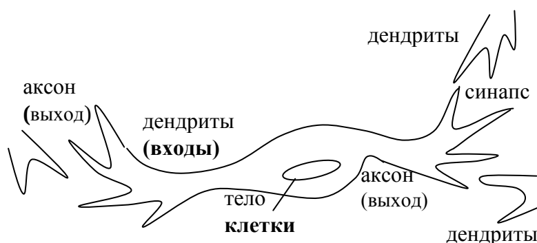
Рис.2. Биологический нейрон
