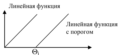
Рис.6. График линейной функции
