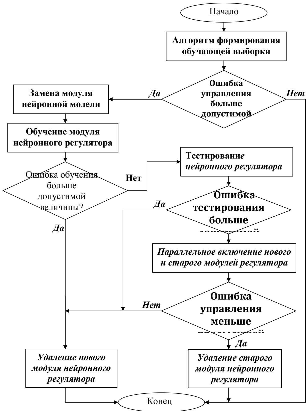
Рис. 16. Алгоритм функционирования адаптивной системы управления с нейронным регулятором
