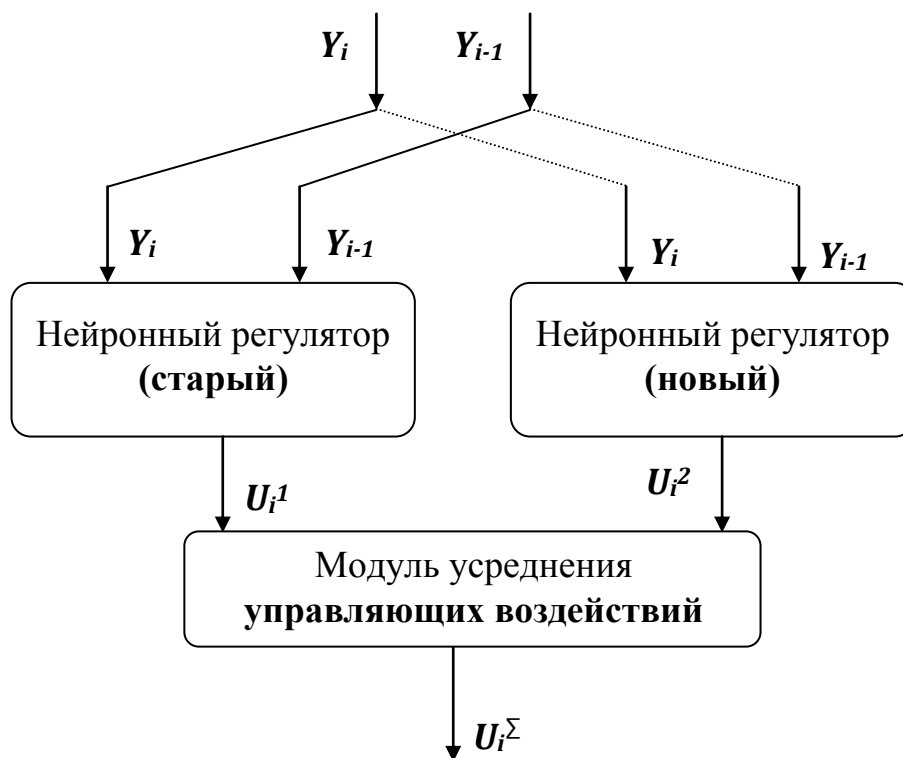
Рис.18. Структурная схема для обеспечения плавного перехода при смене модуля нейронного регулятора
