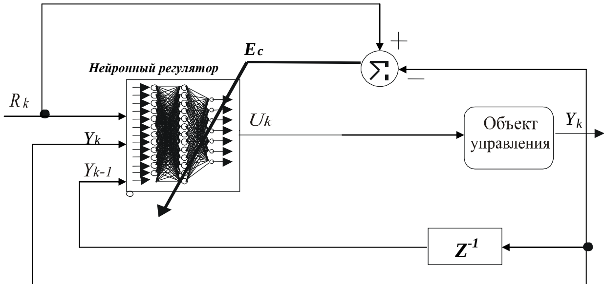
Рис. 13. Структурная схема с опорной моделью эталонного переходного процесса
