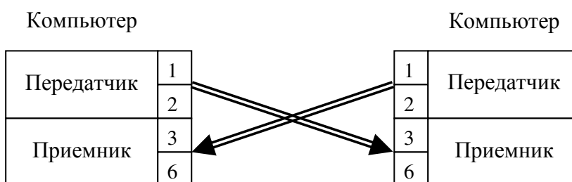
Рис. 1.8. Соединение Компьютер – Компьютер
