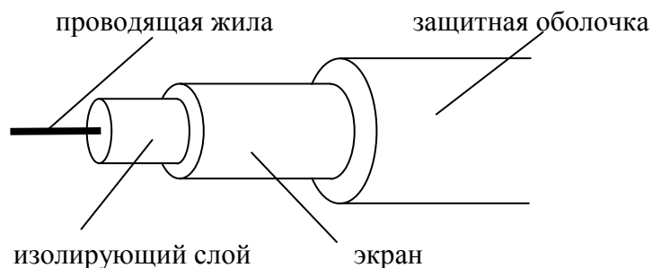
Рис. 1.3. Коаксиальный кабель
