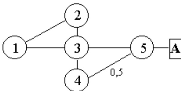
Рис 4.4. Пример EIGRP-системы
