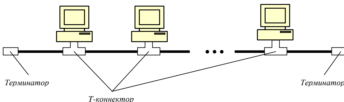
Рис. 1.12. Топология «шина»
