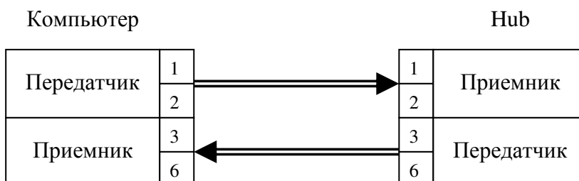
Рис. 1.7. Соединение Компьютер – Hub
