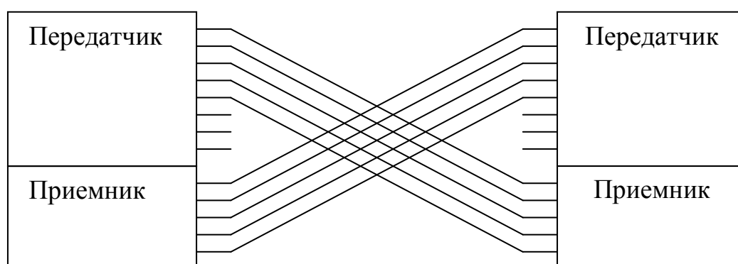
Рис. 2.7. Соединение двух компьютеров по LPT
