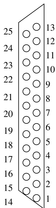
Рис. 2.6. Внешний вид LPT -разъема (со стороны компьютера)
