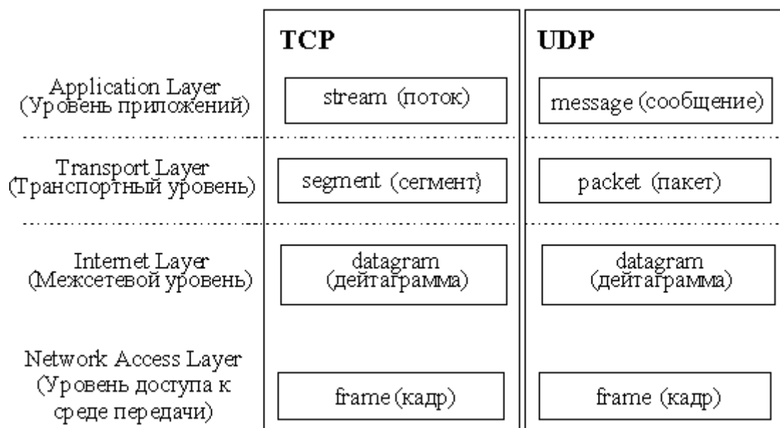
Рис. 5.2. Стек протоколов TCP/IP
