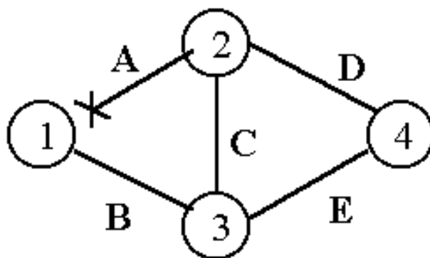
Рис. 4.6. Изменение состояния RIP-системы
