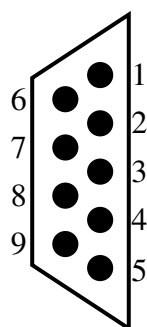
Рис. 2.1. Внешний вид COM-разъема (со стороны компьютера)
