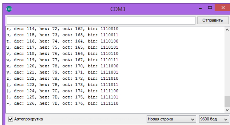
Рис. 2.5. Serial Monitor
