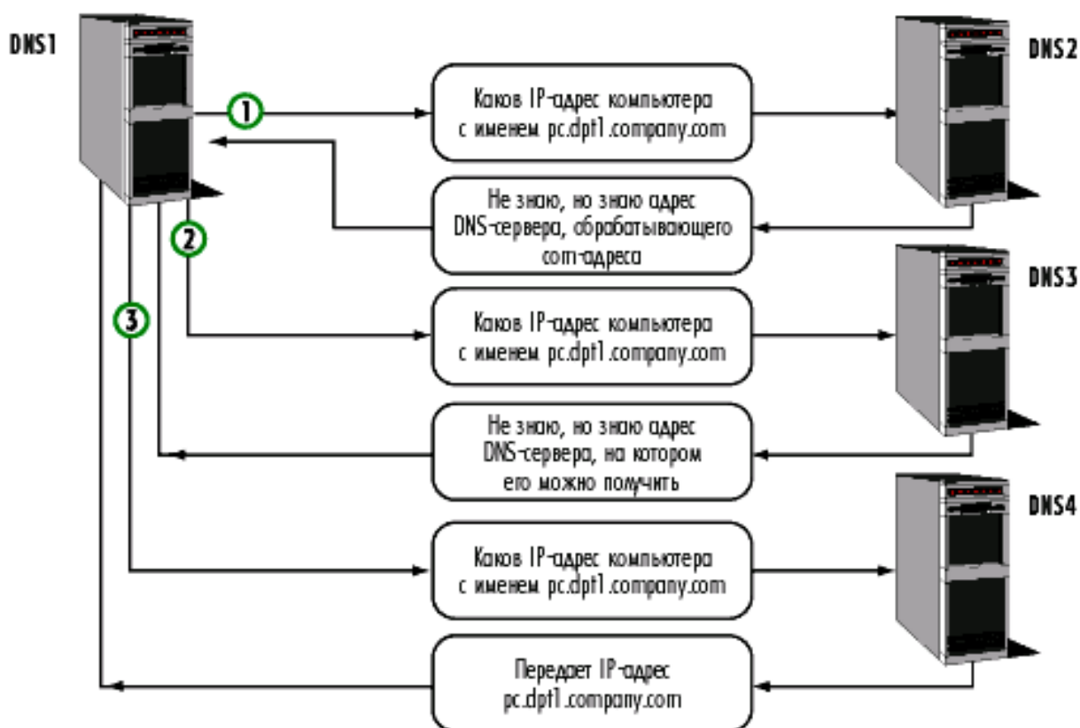
Рис. 3.4. Поиск DNS-сервера
