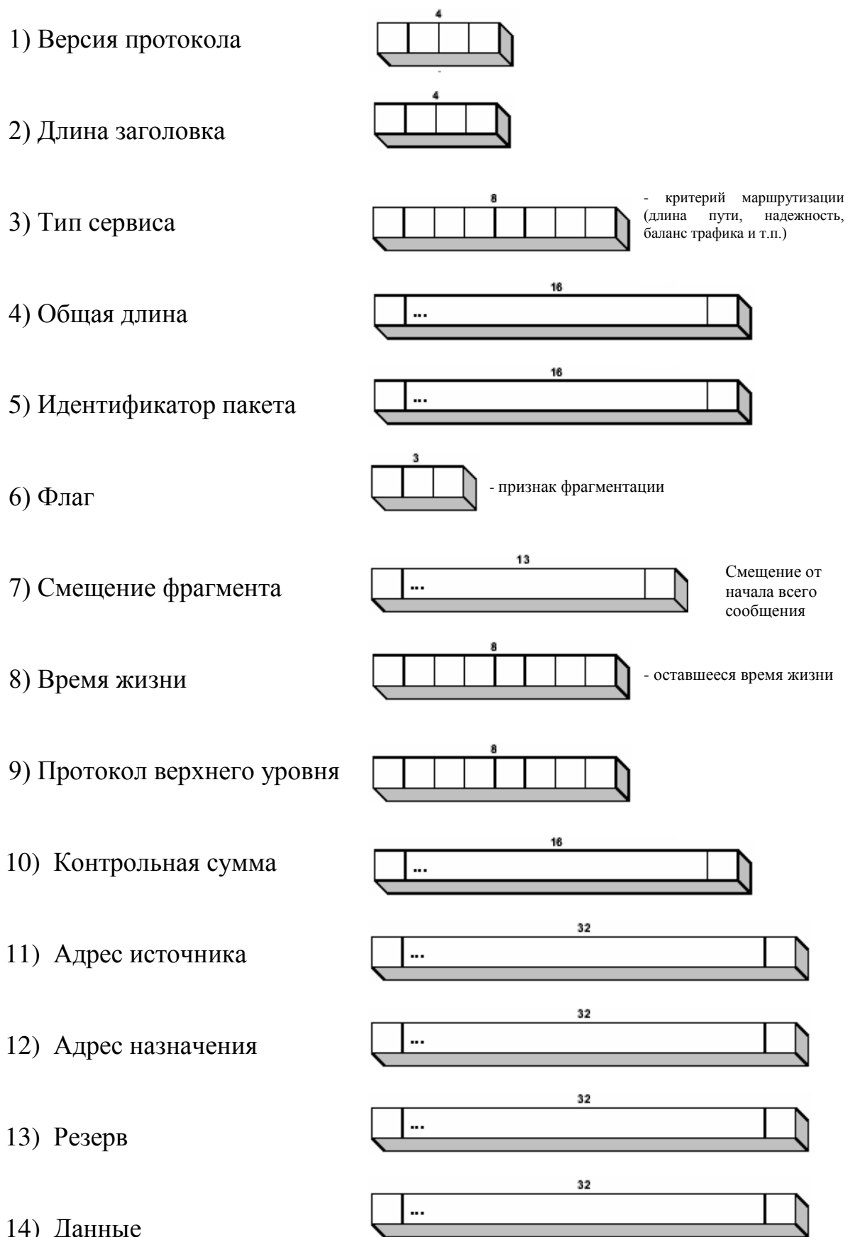
Рис. 4.1. Структура пакета протокола IP
