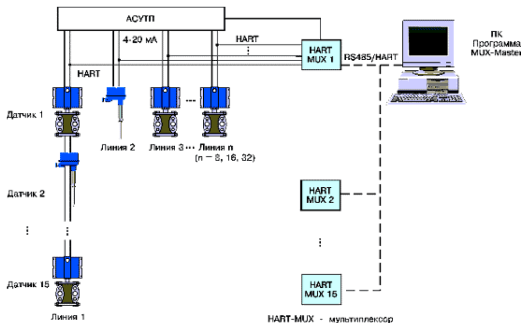
Рис. 6.4. Структурная схема работы мультиплексора
