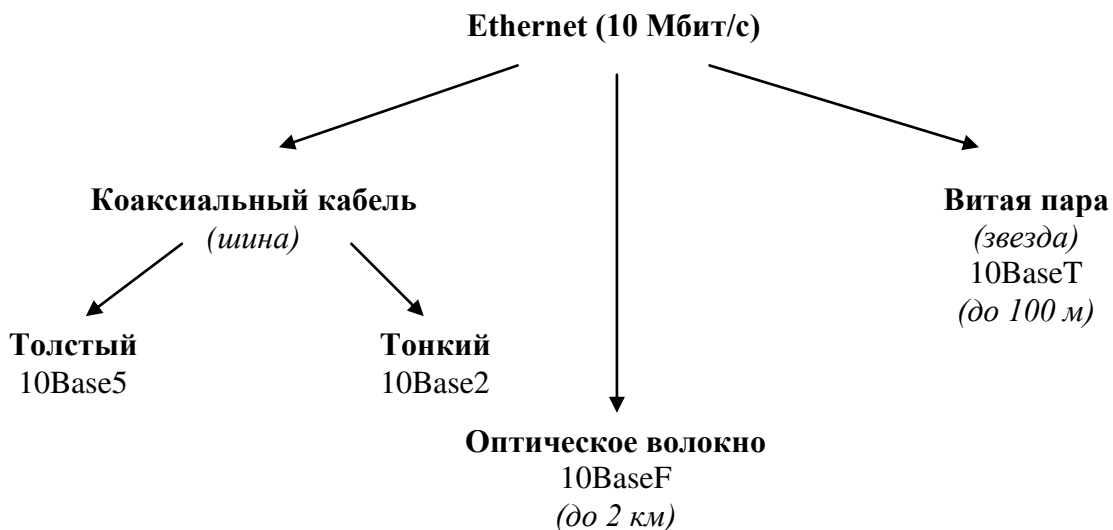
Рис. 1.1. Структура Ethernet 10 Мбит/с
