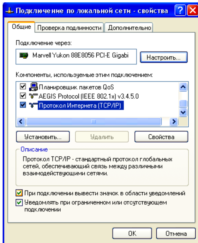
Рис. 1.21. Свойства подключения
