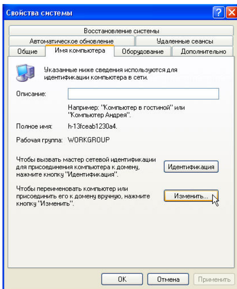
Рис. 1.18. Свойства системы
