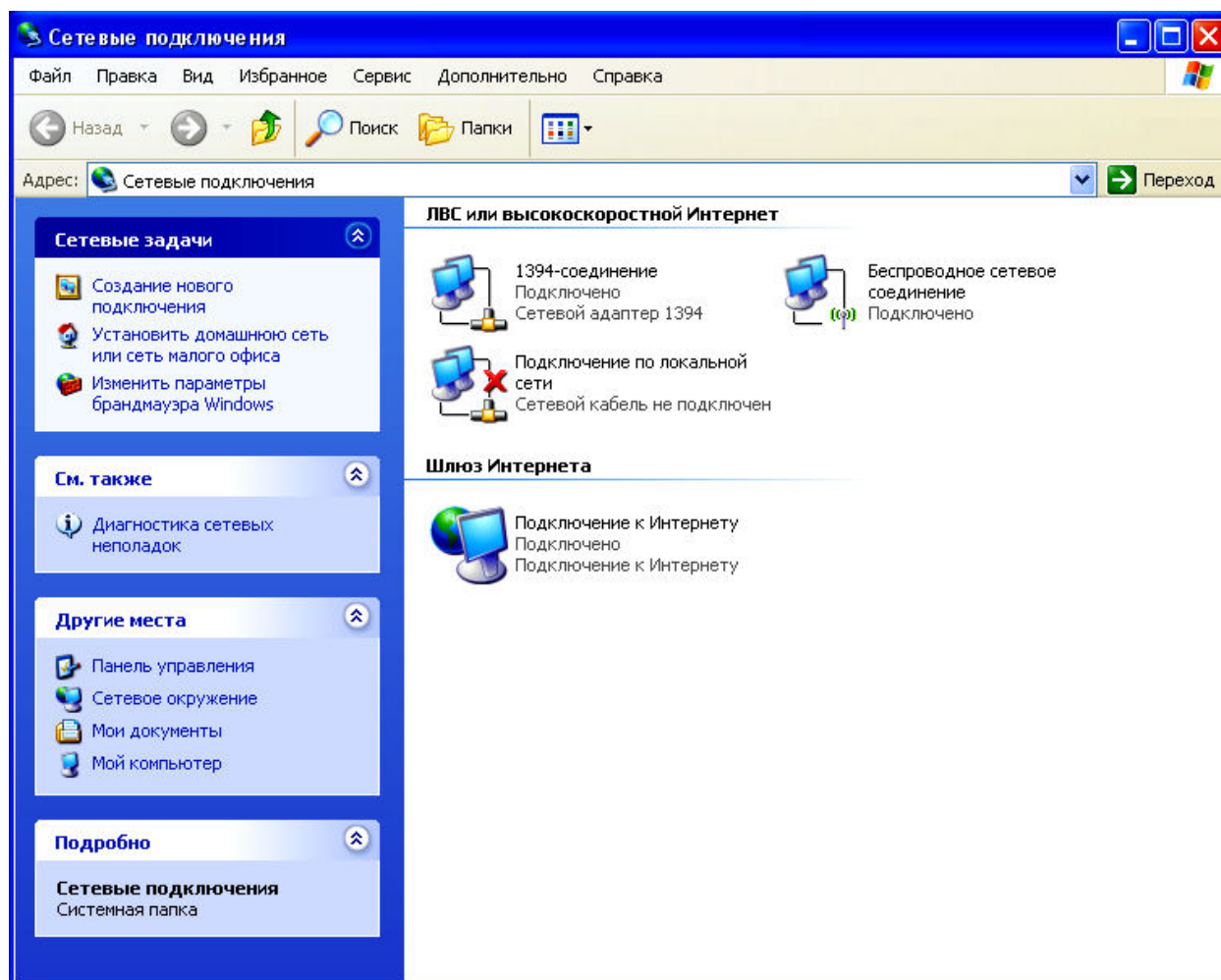
Рис. 1.20. Сетевые подключения
