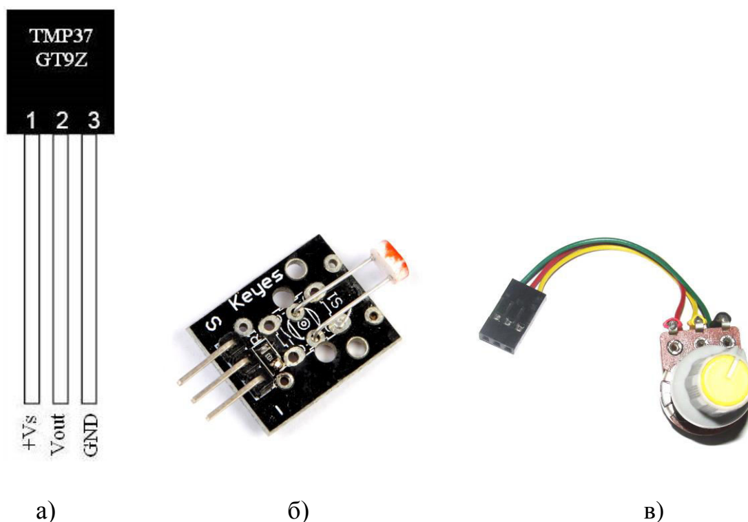
Рис. 2.9. Аналоговые датчики: а) датчик температуры; б) фоторезистор; в) потенциометр
