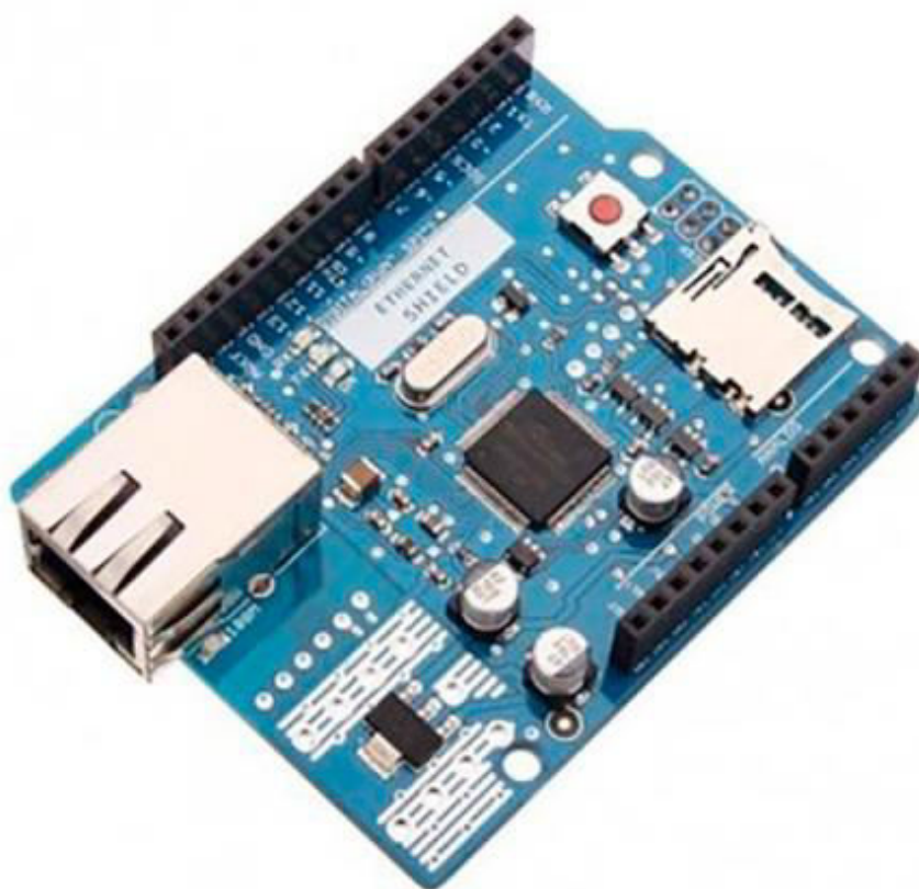
Рис. 2.8. Микроконтроллер Arduino Ethernet Shield
