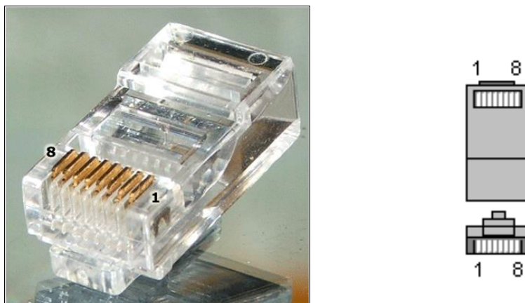
Рис. 1.5. Коннектор RJ-45
