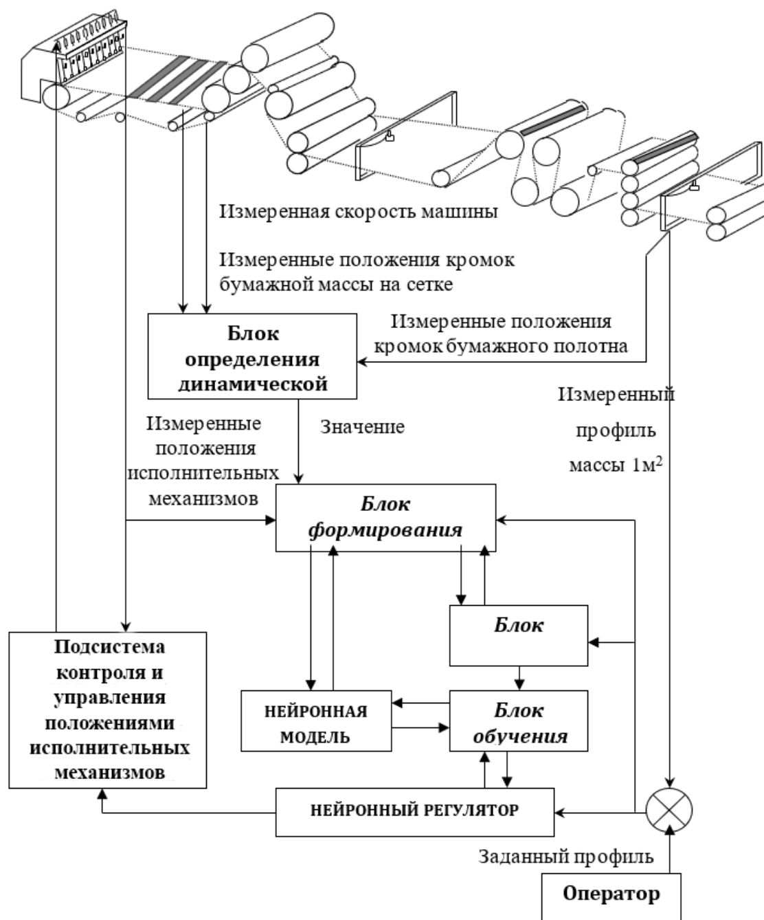
Рисунок 15 – Схема нейросетевой системы управления массой 1 \text{ м}^2 бумаги
