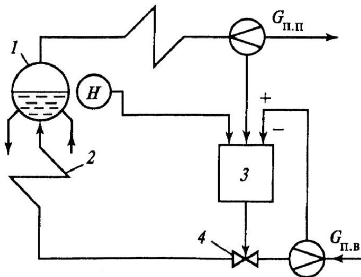
Трехимпульсная АСР питания водой барабанного парогенератора: 1-барабан; 2-водяной экономайзер; 3-регулятор питания; 4-регулирующий клапан питательной воды
