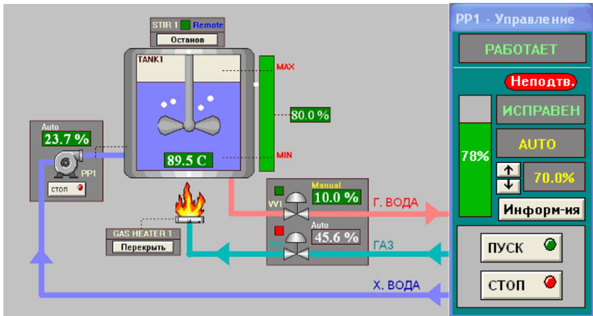
Рис. 5. Схема информационной модели интерфейса «Нагрев горячей воды»
