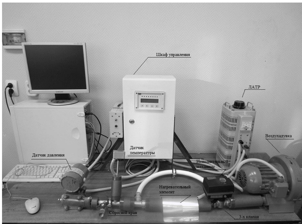
Рис.20. Внешний вид стенда
