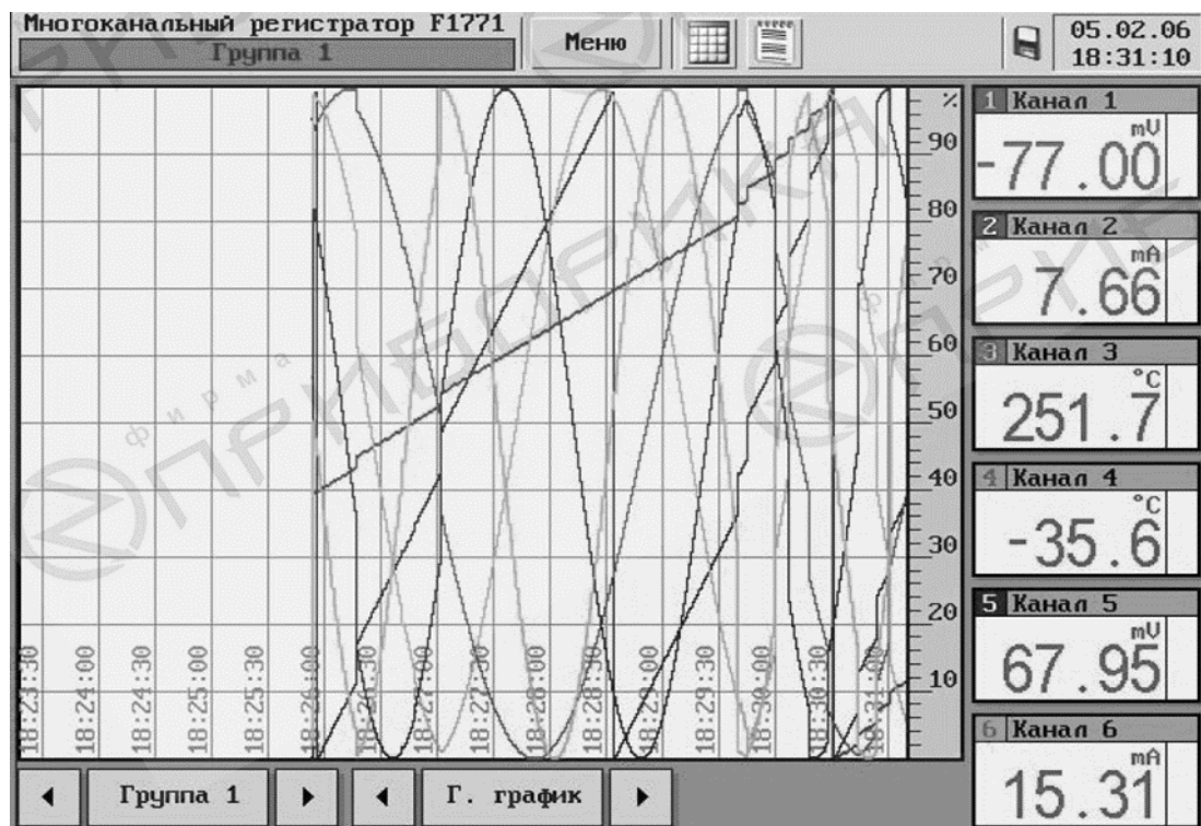
Рис. 27. Внешний вид горизонтального графика
