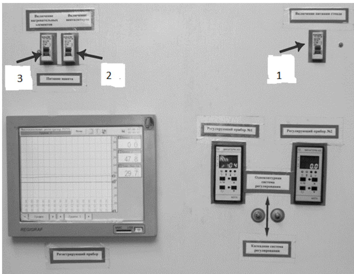
Рис 23. Внешний вид щита управления
