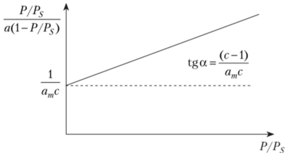
Рисунок 4. Изотерма адсорбции в координатах уравнения БЭТ
