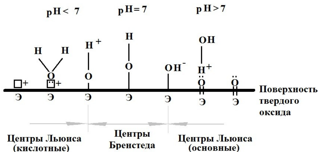
Рисунок 1. Распределение активных центров на поверхности твердого оксида по силе ионизации и кислотно-основным свойствам
