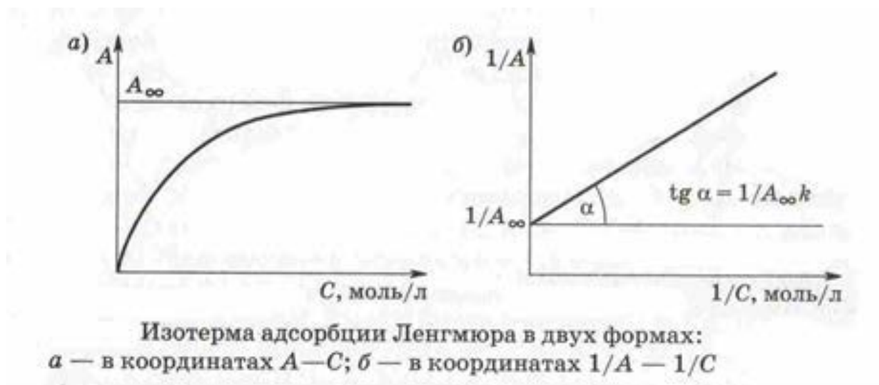
Рисунок 2. Изотерма адсорбции Ленгмюра
