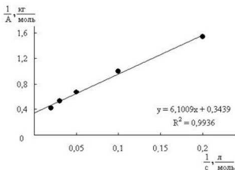
Рисунок 6. Изотерма адсорбции изоамилового спирта в координатах линейной формы уравнения Ленгмюра
