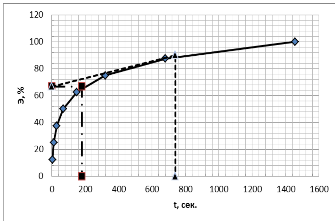
Рис. 4. Зависимость эффективности осаждения от времени
