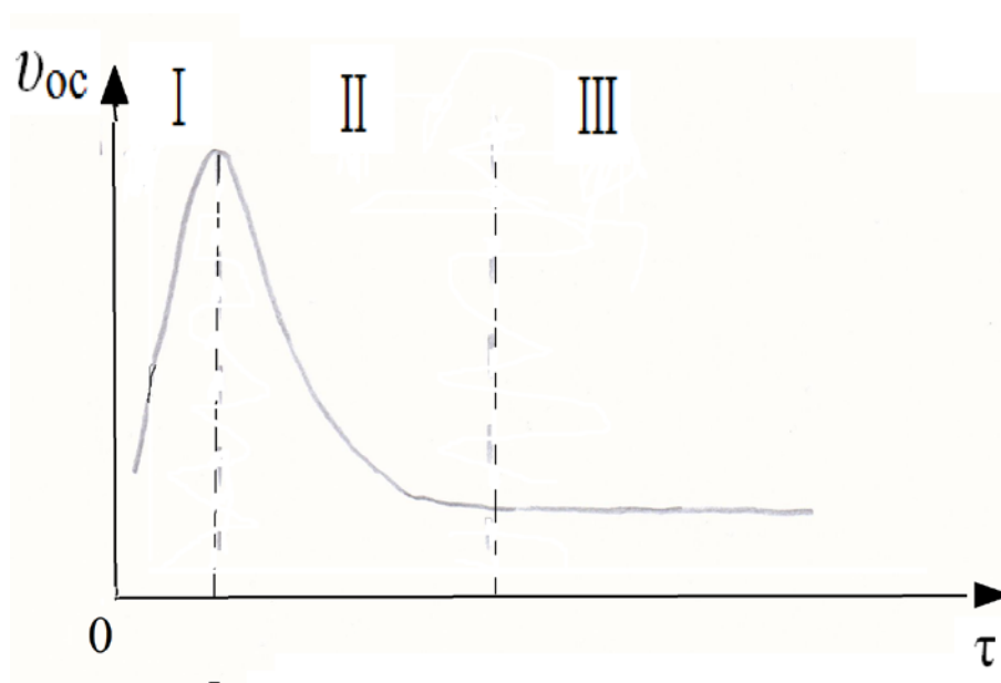
Рис. 1. Кинетика осаждения активного ила:
