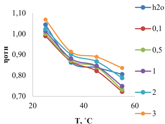
Рисунок 1 – Зависимость относительной вязкости водных систем дикатионной ионной жидкости от температуры
