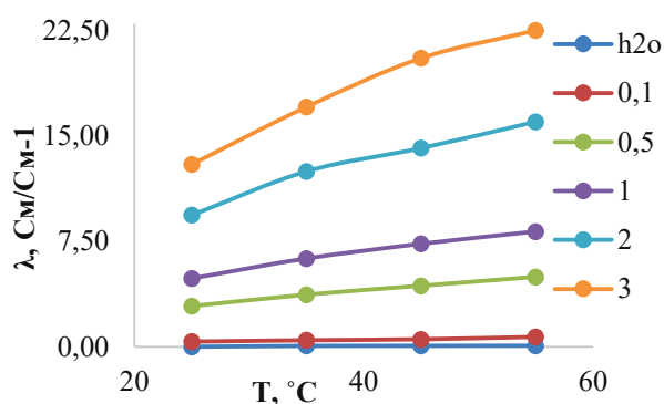
Рисунок 2 – Зависимость электропроводности водных систем ионной дикатионной жидкости от температуры
