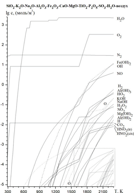
Рисунок 2 – Газовые фазы
