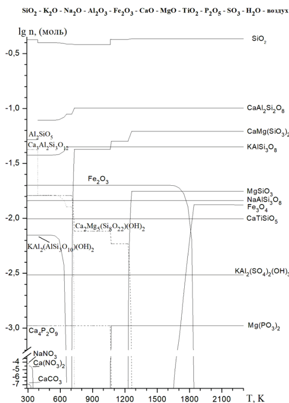
Рисунок 1 – Конденсированные фазы
