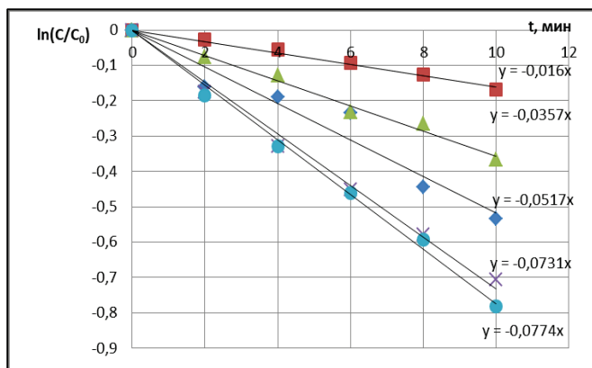
Рисунок 2 – Зависимость \ln(C/C_0)=f(t) для сосуда D = 330 мм и d_m = 142 мм (ромб – 200 об/мин; квадрат – 250 об/мин; треугольник – 300 об/мин; крест – 400 об/мин; круг – 500 об/мин)
