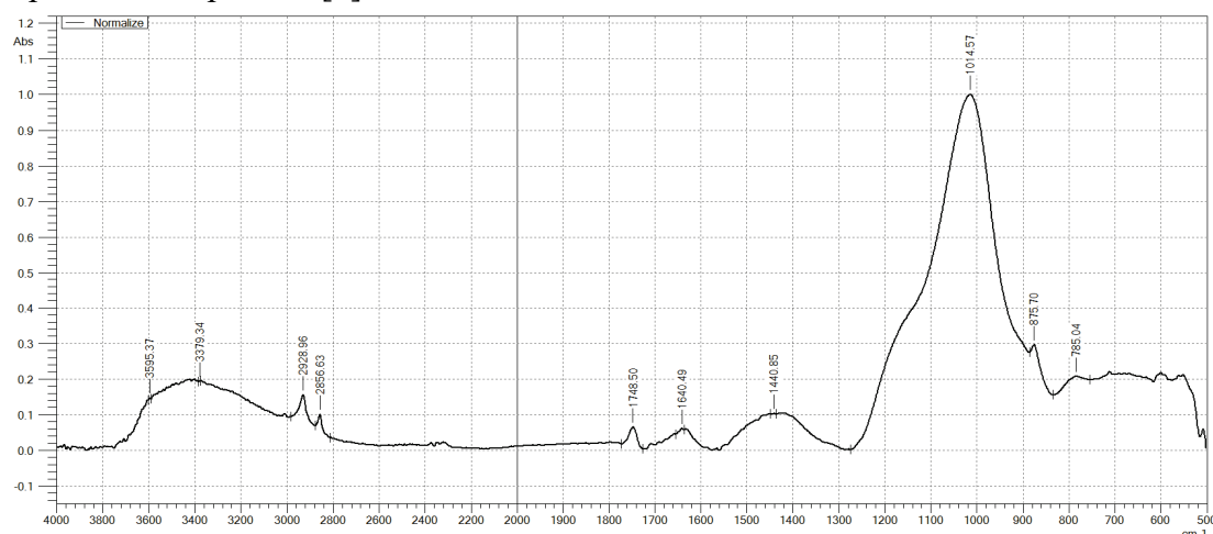
Рисунок 2 – ИК-спектр опытного образца силикагеля
