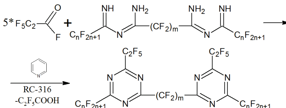
Рисунок 2 – Схема получения перфторированных бистриaziнов
