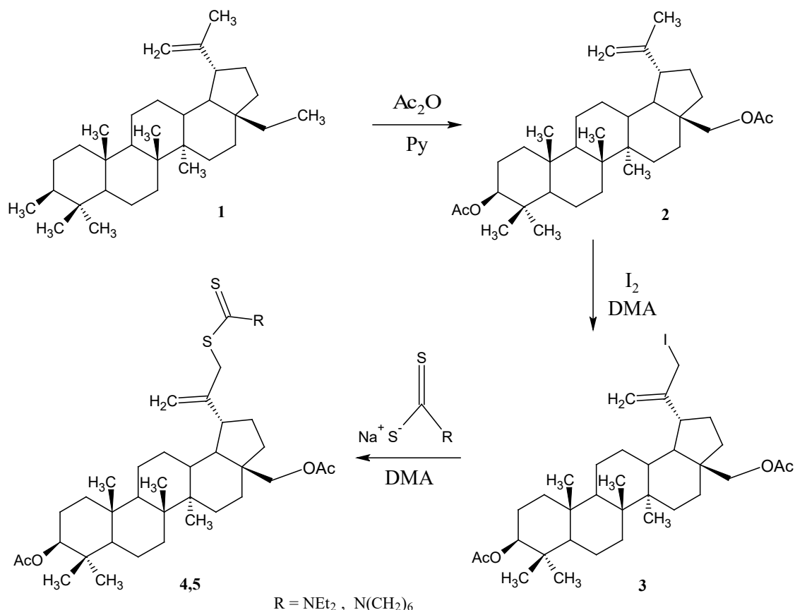
Рисунок – Схема получения 30-(карбонотиоил)сульфанильных производных бетулина
