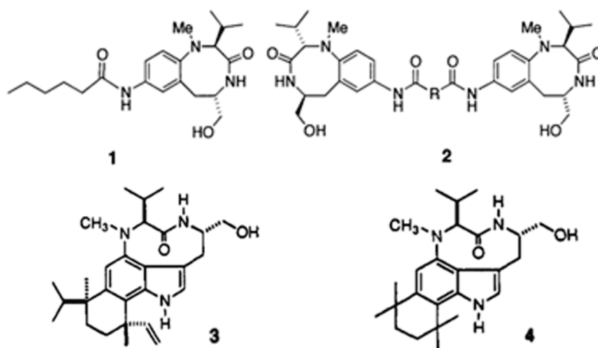
Рисунок 2 – Схема представителей синтетических производных диазонинов
