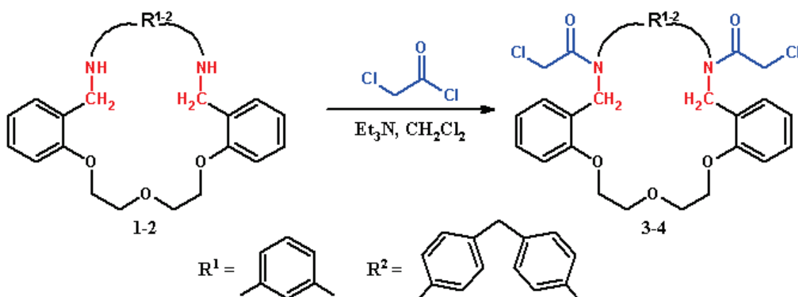
Рисунок 1 – Схема получения N-галогенацилпроизводных N,O-макроциклических соединений 3-4
