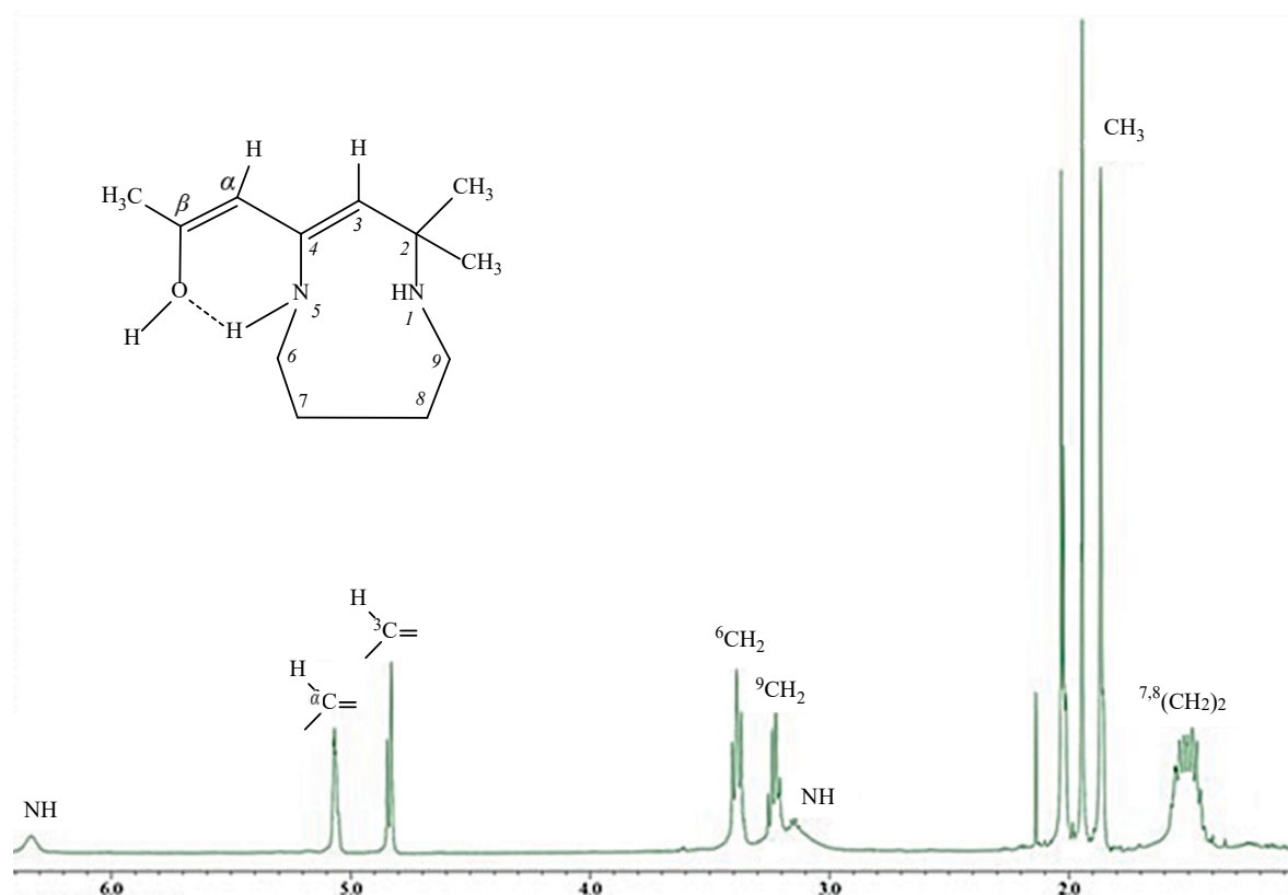
Рисунок 4 – Спектр ЯМР 1 H диазонины IC (в CDCl 3 )
