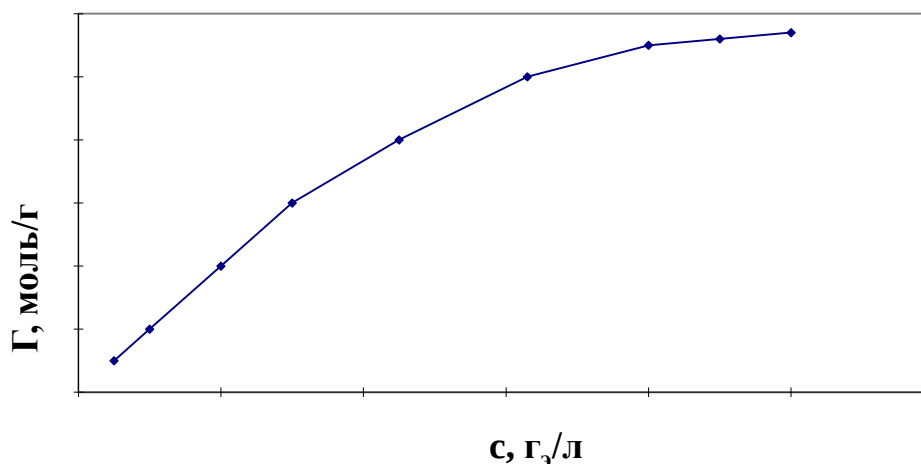
Рис. 2. Зависимость адсорбции от равновесной концентрации кислоты
