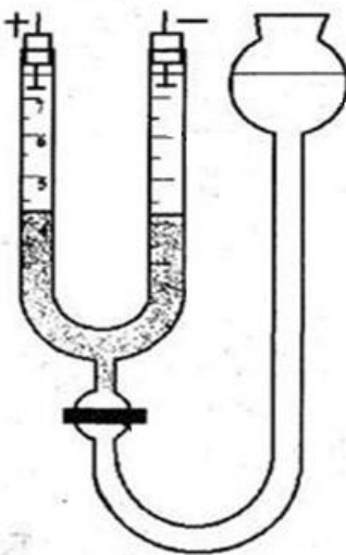
Рис. 3. Схема U-образной трубки для определения \xi -потенциала
