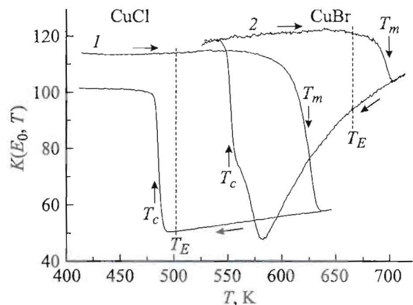
Рис. 3. Зависимость поглощения НК CuCl (1) и CuBr (2) при линейном нагреве до плавления и охлаждении до кристаллизации. Стрелками указаны направления хода температуры и положения температур плавления T_m и кристаллизации T_c . T_E — температуры измерения спектров поглощения НК и НР. Энергия фотонов оптического зонда E_0 = 3.242 (1) и 3.00 eV (2).
