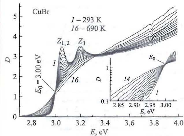
Рис. 2. Температурные изменения в спектрах фундаментального поглощения НК CuBr. На вставке показана длинноволновая часть спектров поглощения в полулогарифмическом масштабе. Температурный шаг составляет около 30 K.
