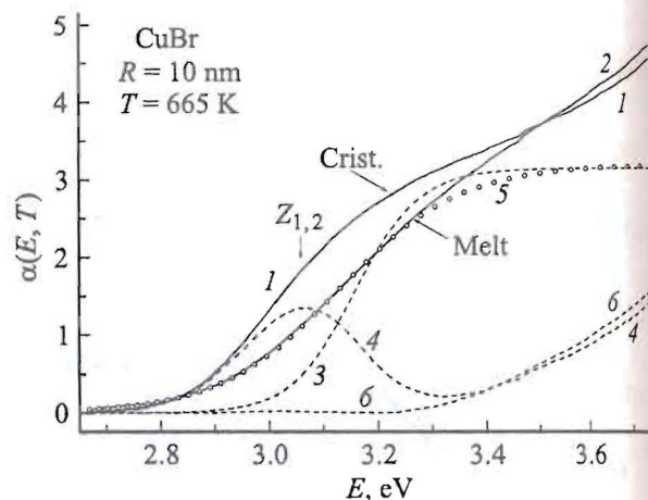
Рис. 5. Спектры фундаментального поглощения частиц CuBr в кристаллическом (1) и расплавленном (2) состояниях. Остальные обозначения те же, что на рис. 4.
