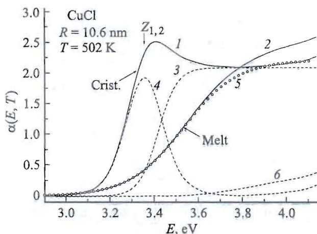
Рис. 4. Спектры фундаментального поглощения частиц CuCl в кристаллическом (1) и расплавленном (2) состояниях. Кривые 3 и 5 — расчет согласно соотношению (2) зона-зонного поглощения НК и расплава соответственно; кривая 4 — экситонное поглощение НК (разность кривых 1 и 3); кривая 6 — поглощение в глубине зона-зонных переходов (разность кривых 2 и 5).
