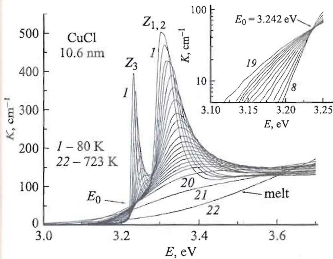
Рис. 1. Спектры фундаментального поглощения НК CuCl со средним радиусом 10.6 nm. На вставке показана длинноволновая часть спектров в полулогарифмическом масштабе. Кривая 20 — начало плавления, кривая 22 — спектр нанорасплава.
