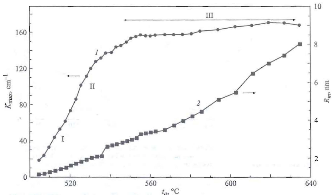
Рис. 2. Зависимости оптического поглощения при энергии E_0 (1) и среднего радиуса R_m ансамбля частиц CuCl (2) от температуры t_a образования фазы CuCl в образце стекла при времени выдержки 3 h.
