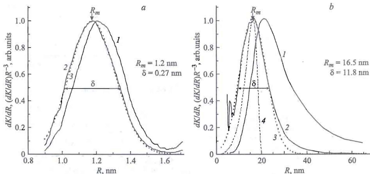
Рис. 4. Распределение нанокристаллов CuCl по объему dK/dR (1) и по радиусу (dK/dR)R^{-3} (2) для участка образца с температурой отжига 500 (а) и 720°C (b). Кривые 3 (пунктир) представляют аппроксимацию кривых 2 распределениями Гаусса с шириной распределения \delta = 2s . Кривая 4 — распределение Лифшица-Слезова.
