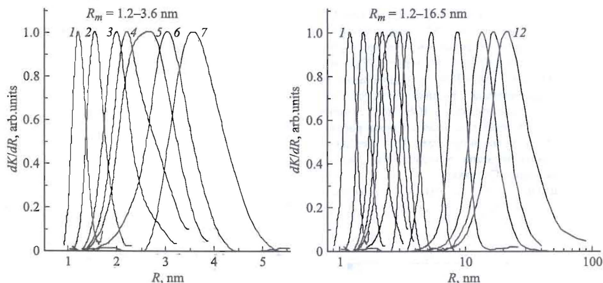
Рис. 5. Изменение формы распределения частиц CuCl по объему на различных участках образца стекла. Температура отжига изменялась вдоль образца от 500 (1) до 710°C (12).
