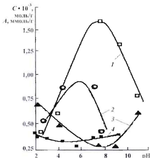
Рис. 4. Зависимость параметров A (1, 2) и C (3, 4) при сорбции из 0,10 М (1, 3) и 0,25 М (2, 4) растворов глицерина от pH
