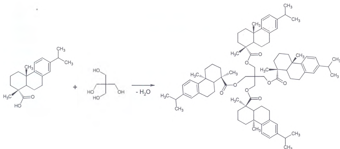
Рис. 3. Схема синтеза тетраэфира пентаэритрита и дегидроабиетиновой кислоты
