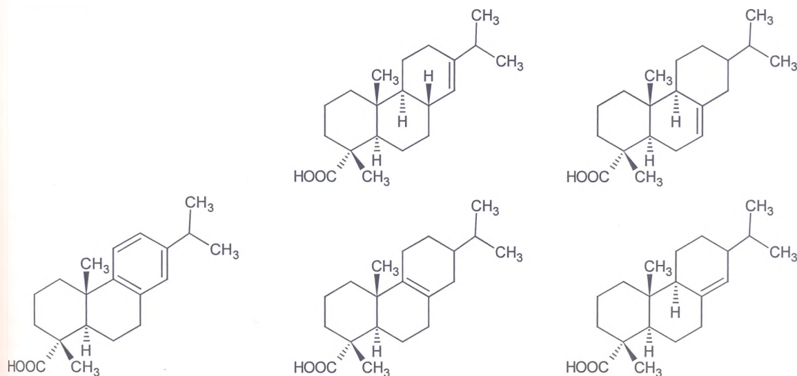
Дегидроабиетиновая кислота
