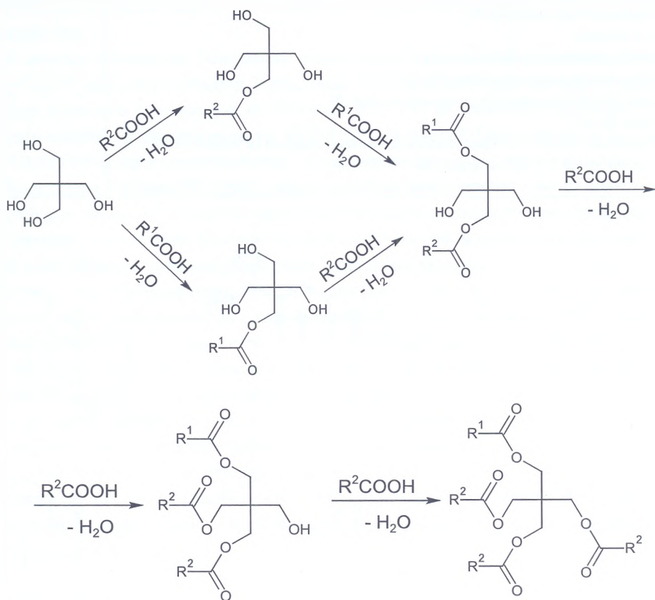
Рис. 2. Схема образования моно-, ди-, три- и тетраэфиров пентаэритрита и смоляных кислот ( \text{R}^1 и \text{R}^2 – остатки дегидроабетиновой и дигидроабетиновых кислот)
