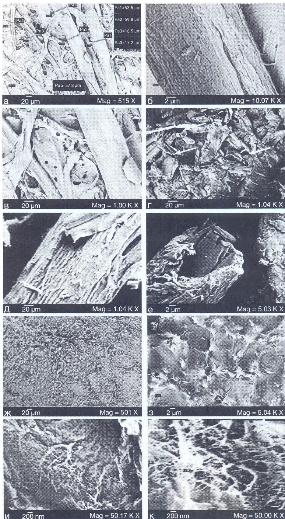
Рис. 4. СЭМ фотографии поверхности исходного образца бумаги (а, б, в) и целлюлозных материалов, полученных из бумаги: ПЦ (г, д, е), ГГ Г-4 (ж, з), ЛФГ Г-4 (и) и ЛФГ Г-3 (к). Обозначения: 4 (а) – приведены диаметры волокон, 4 (г) – указаны поры (размер 1–2 \mu\text{m} – стрелки красного цвета; сквозные отверстия – стрелки белого цвета)
