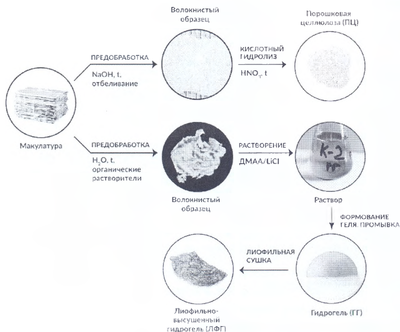
Рис. 2. Схема получения порошковых целлюлоз, гидрогелей и лиофильно-высушенных гидрогелей из бумажной макулатуры
