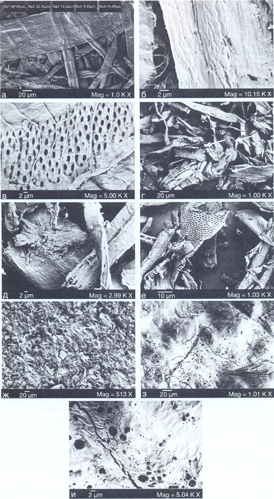
Рис. 5. СЭМ фотографии поверхности исходного образца картона (а, б, в), и целлюлозных материалов, полученных из него: ПЦ (г, д, е), ГГ К-2 (ж), ЛФГ К-2 (з, и). Обозначения: 5 (а) – приведены диаметры волокон; 5 (г) – указаны сквозные отверстия
